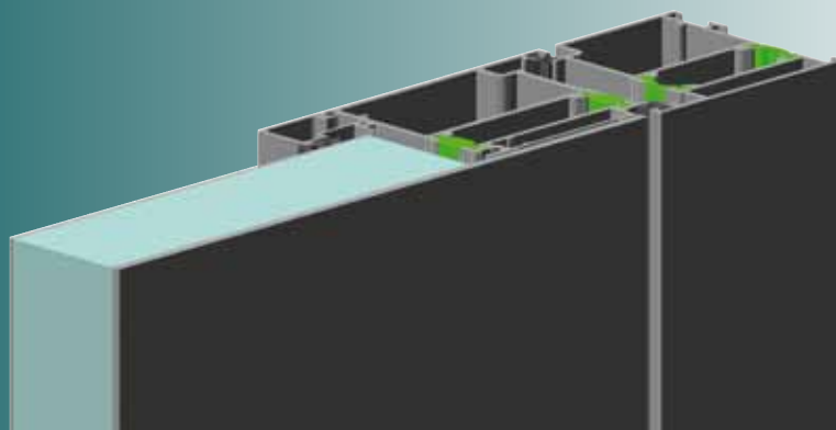
einseitig flügelüberdeckende Füllung
